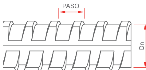
Sección Longitudinal
