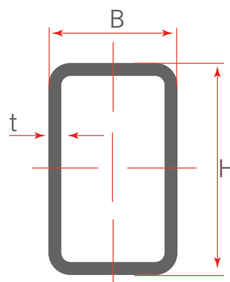
Tubería Mecánica Rectangular
